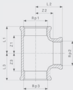
T-Stück - Rotguss oder Siliziumbronze Modell 3130
