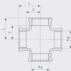
Kreuzstück - Rotguss oder Siliziumbronze Modell 3180
