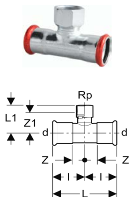
T-Stück mit I.G. Abgang
