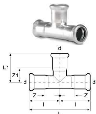
Red.T-Stück
