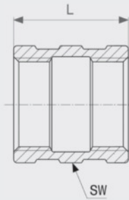
Muffe - Rotguss oder Siliziumbronze Modell 3270
