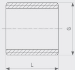
Nippel - Rotguss oder Siliziumbronze Modell 3531
