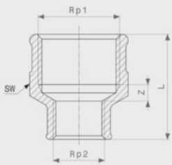
Reduziermuffe - Rotguss oder Siliziumbronze Modell 3240
